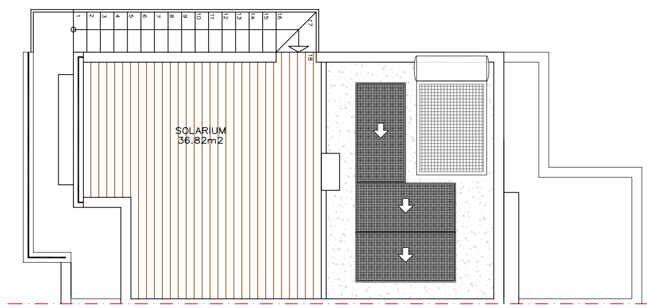
PLANTA CUBIERTAS
