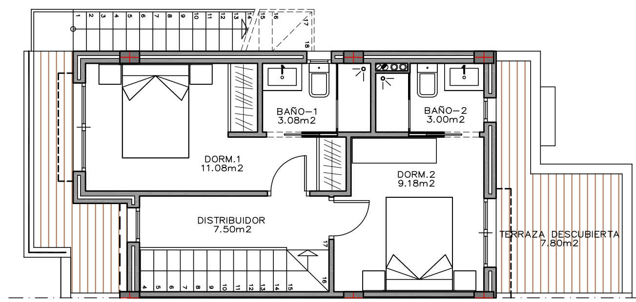
PLANTA PRIMERA
