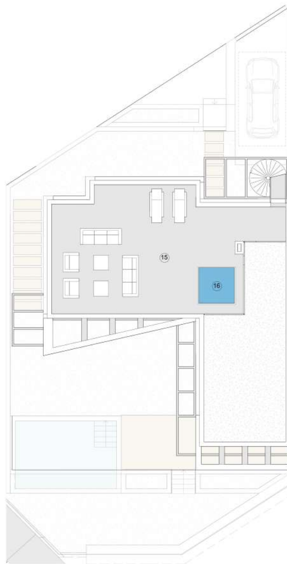
PLANTA PRIMERA / FIRST FLOOR
