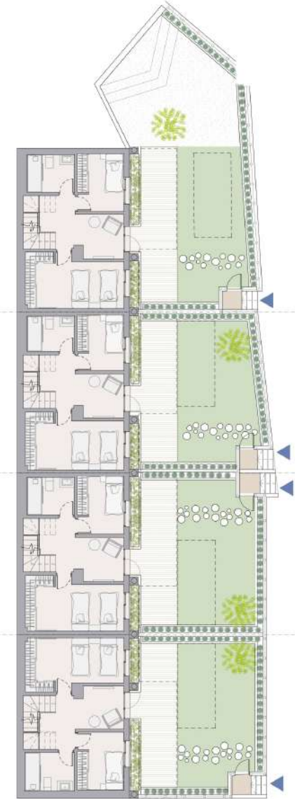
Planta / Floor Inferior
