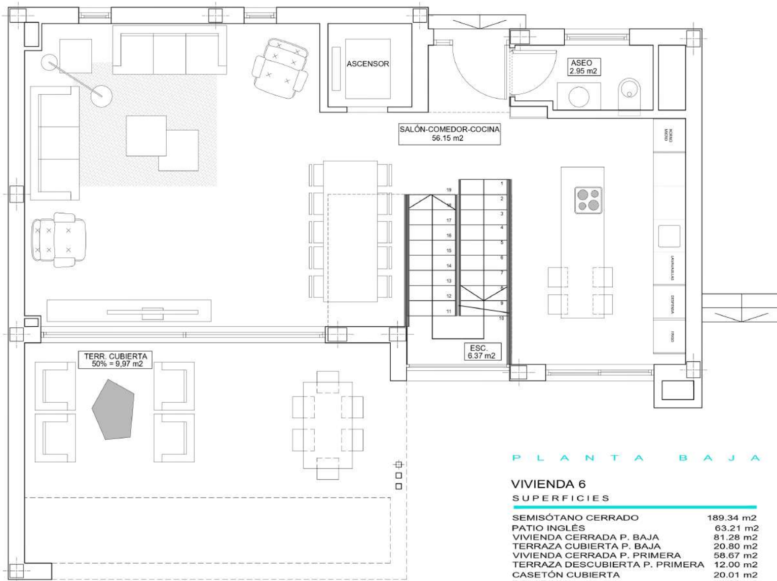
PLANTA BAJA
