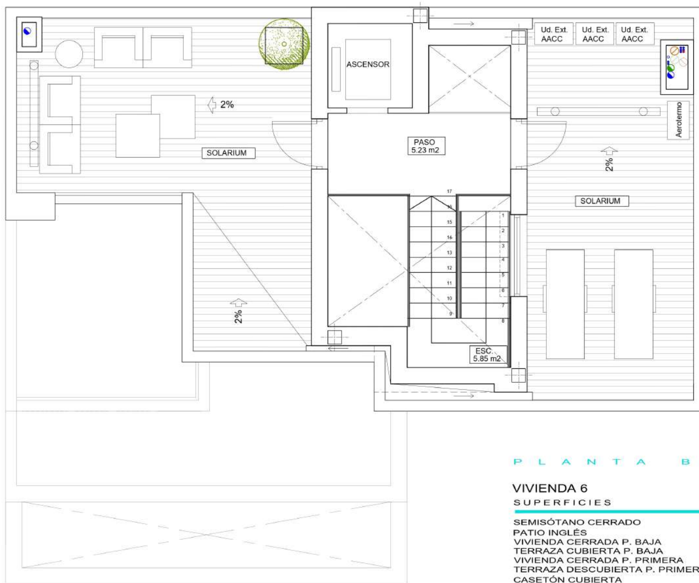
PLANTA SOLARIUM
