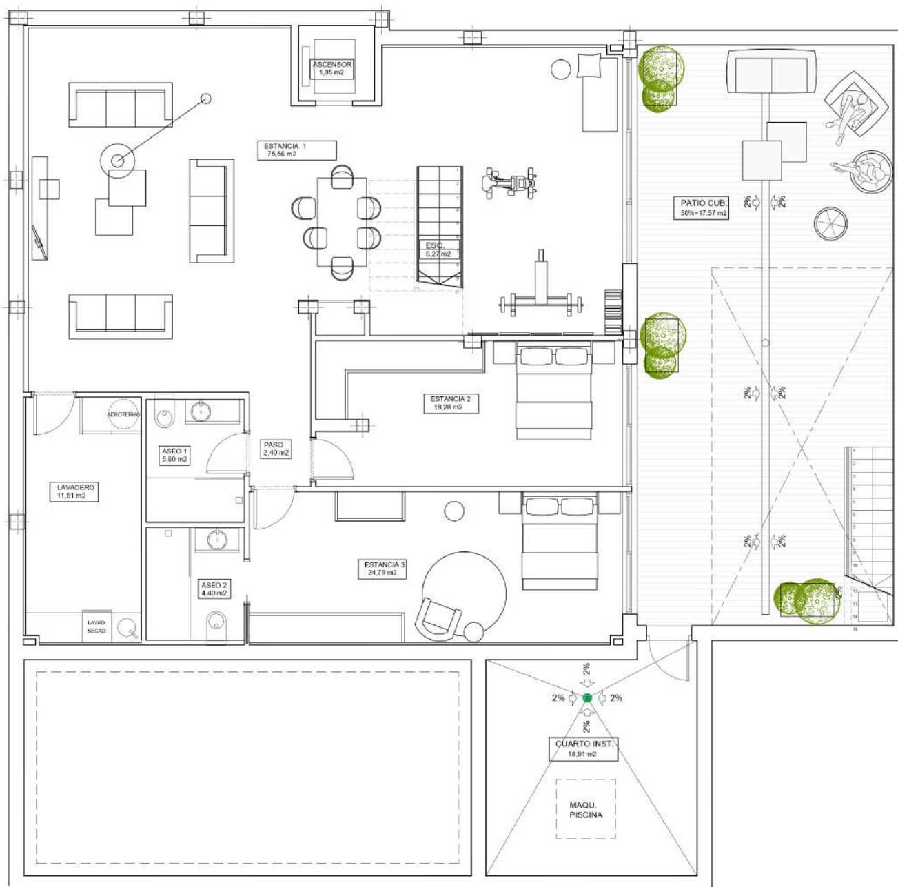
PLANTA SÓTANO VIV. 6
