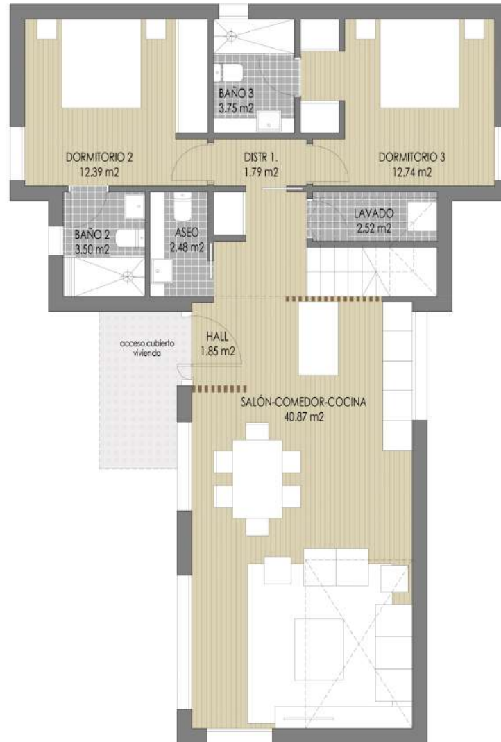
PLANTA BAJA
