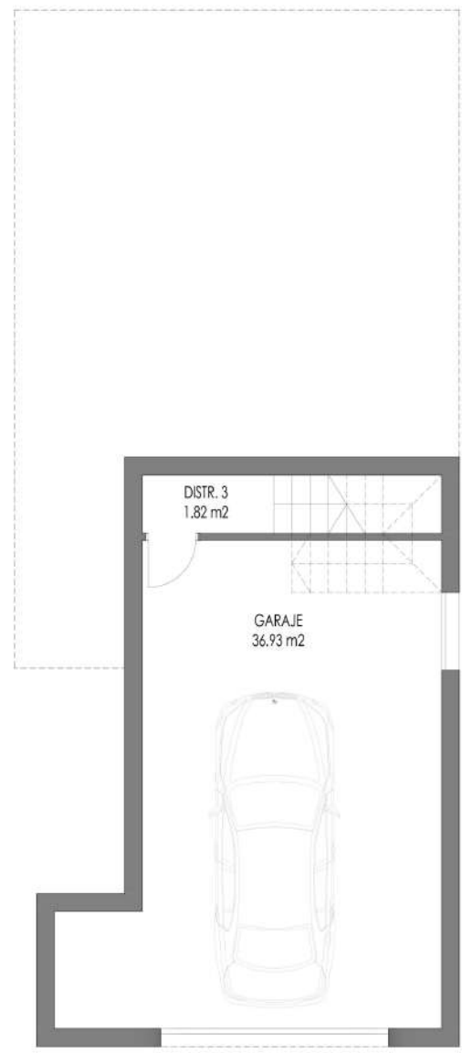
PLANTA SÓTANO
