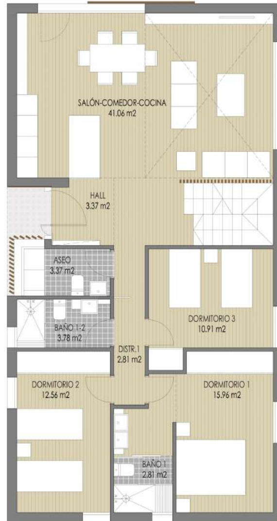
PLANTA BAJA
